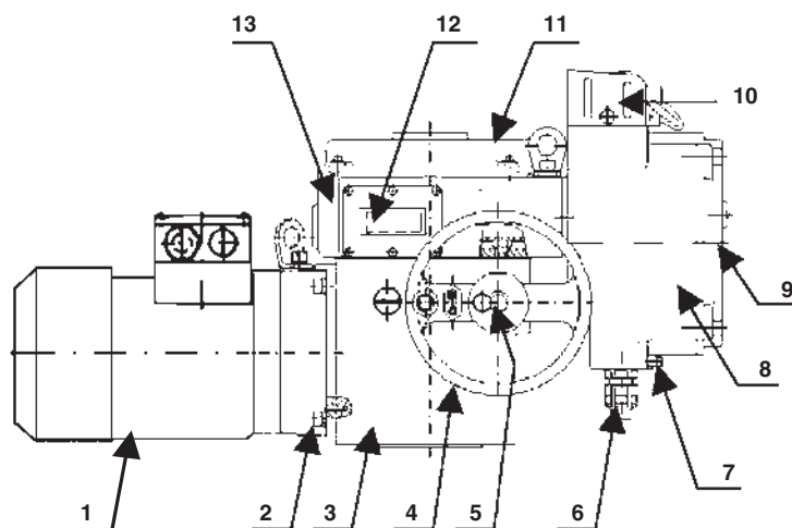
Sestava servomotoru (s elektronickým systémem DMS2 ED)
